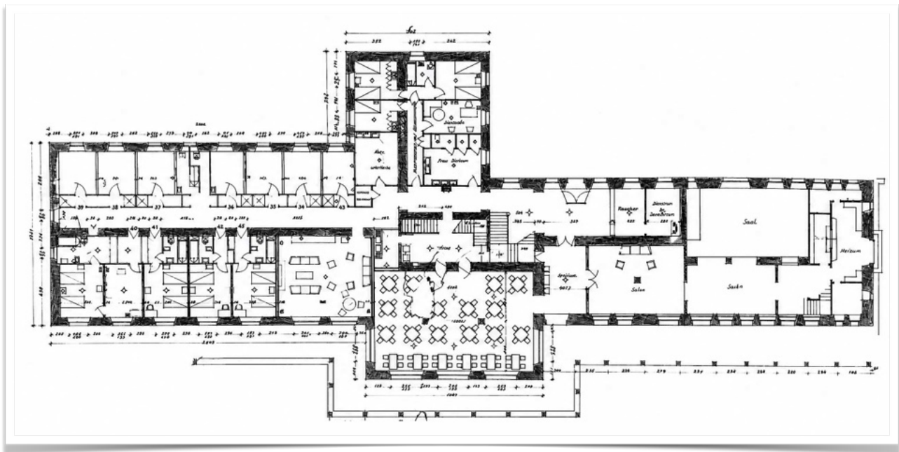
8503 1945. Plano de la II ampliación trazada por Julián Delgado Úbeda y José María Muguruza Otaño.
