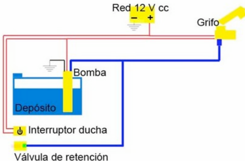
ESQUEMA ORIGINAL WESTFALIA AGUA FRÍA
